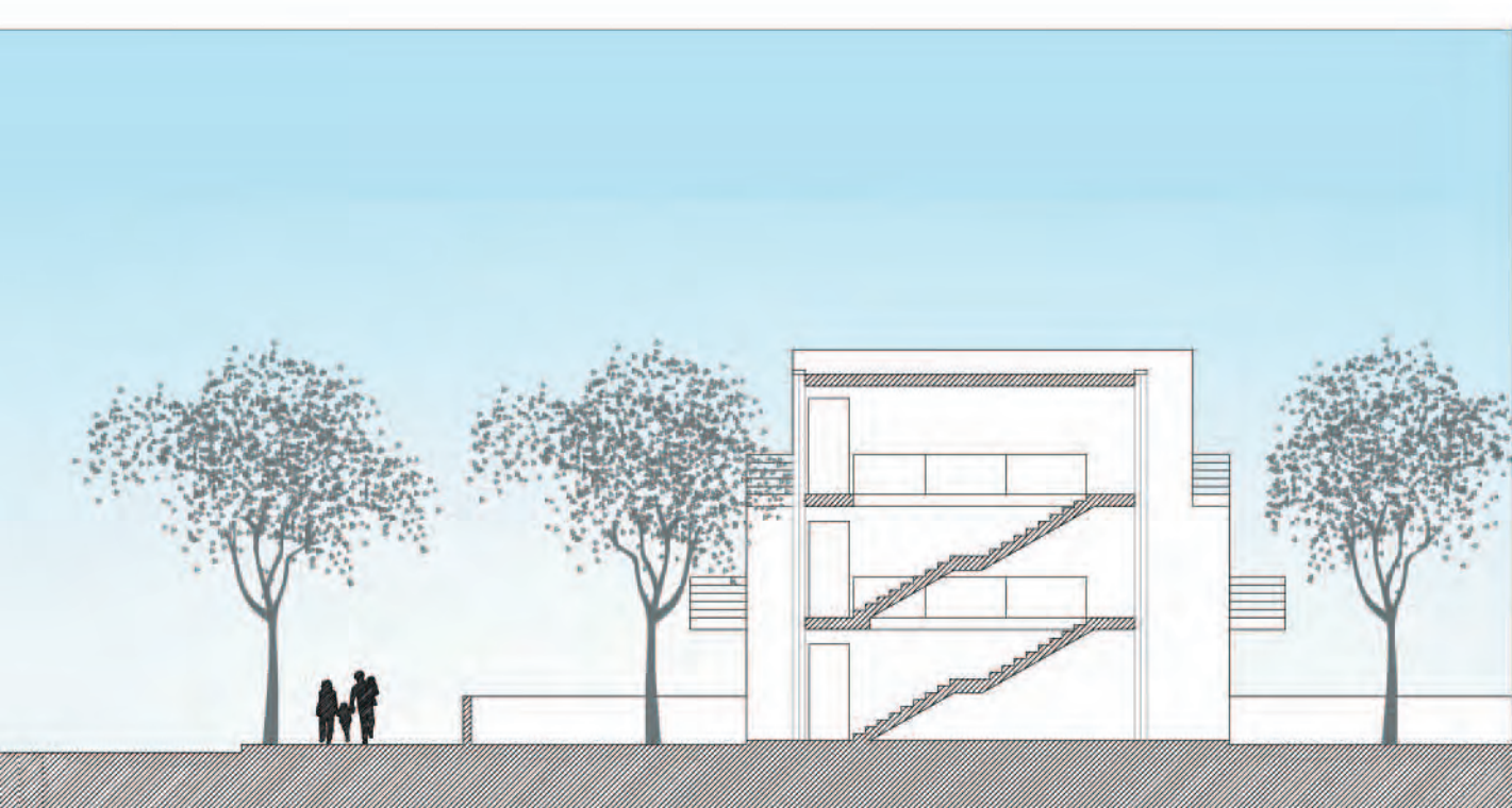
Sezione A-B
