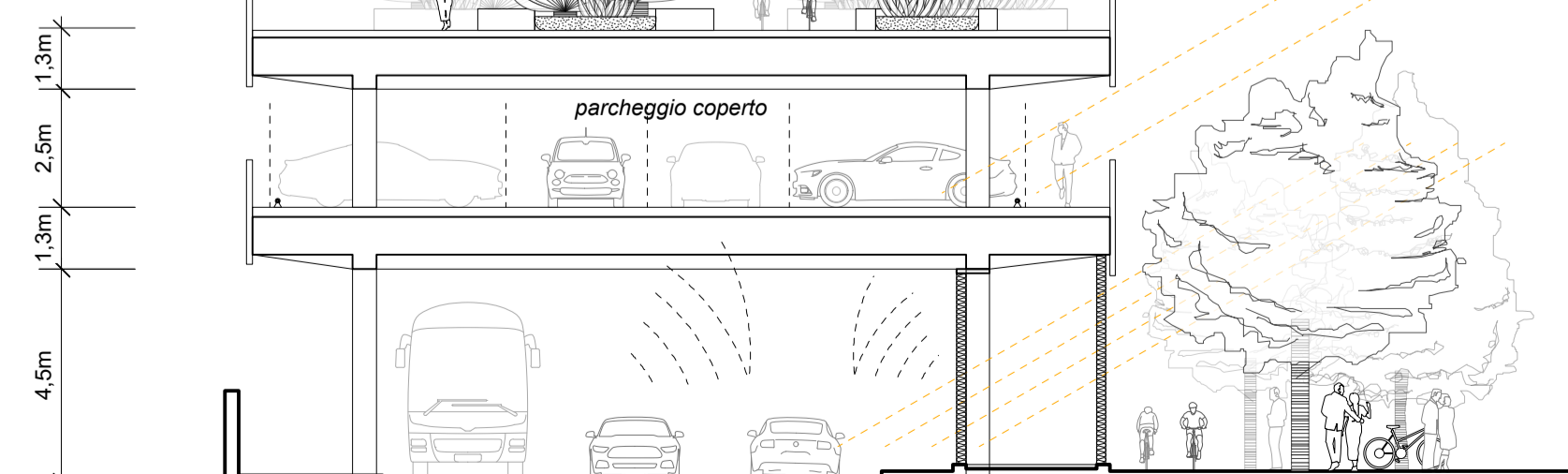
sezione tipologica di progetto
